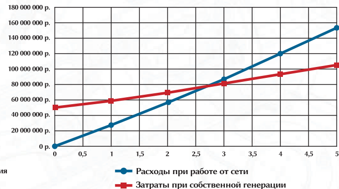
Срок окупаемости ГПТЭС 1 МВт с объемом инвестиций 50 млн. руб. примерно 2,5 года
